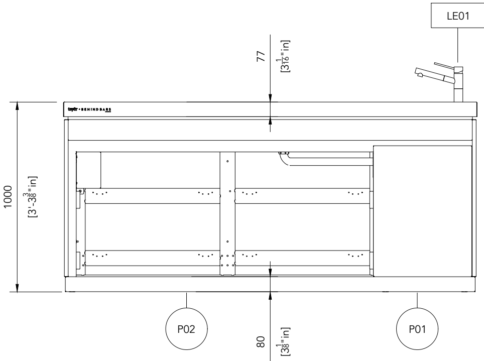
ELEVATION A
