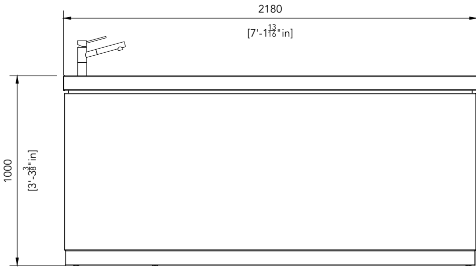
ELEVATION B
