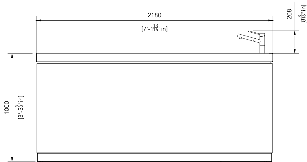
ELEVATION B
