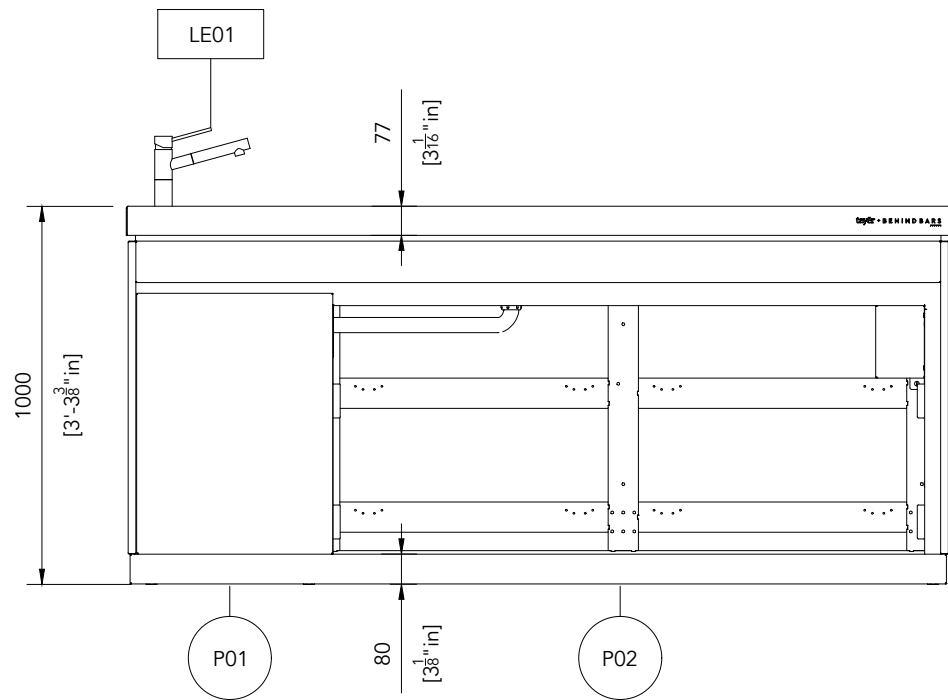
ELEVATION A
