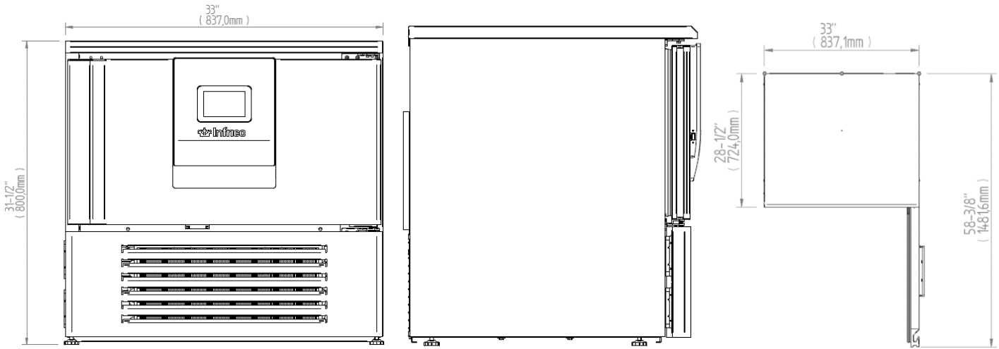
ELEVATION
