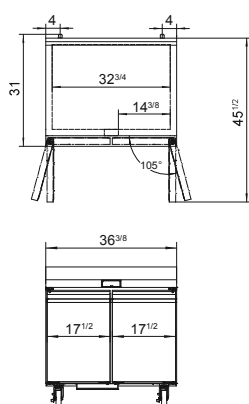
AWR36SD / AWF36SD
